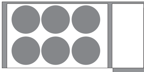
Keykeg 10+20L Slimkeg 20L Ø 237mm
